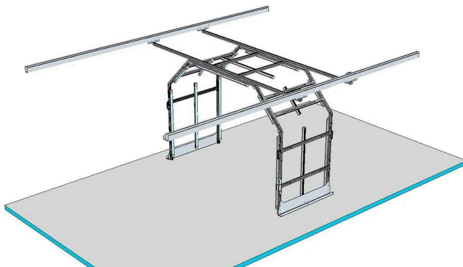
Impianto arco aereo in versione completa Overhead arch on rails
