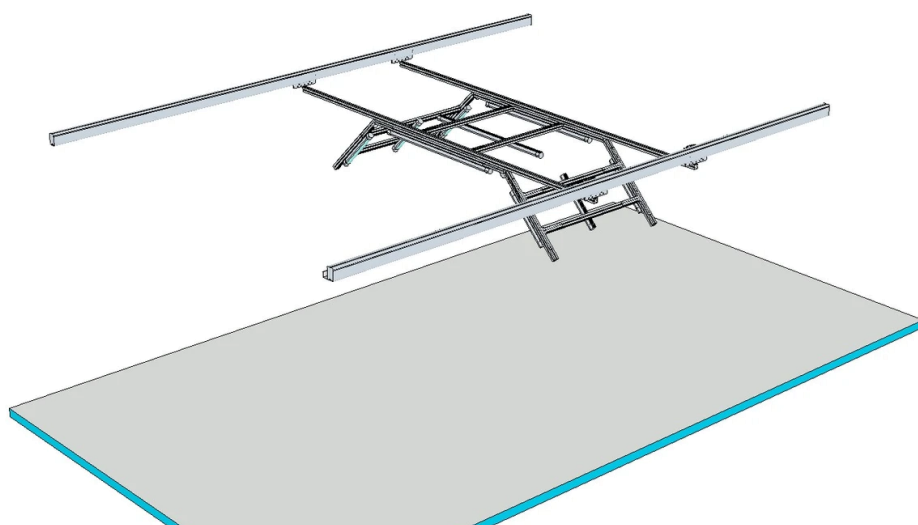
Impianto arco aereo in versione snella Overhead arch-slim version
